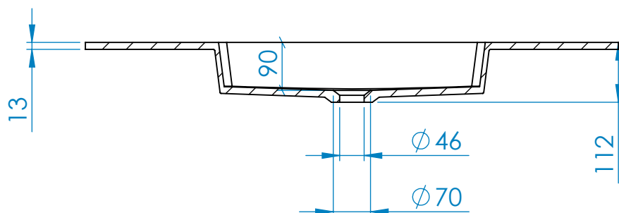
SECCIÓN A-A
