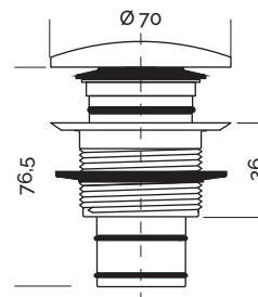
Válvula clic-clac Dolotek (mm)
