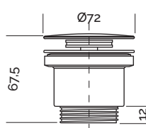
Válvula de salida libre cromo (mm)
