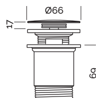
Válvula clic-clac con rebosadero cromo (mm)
