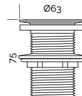
Válvula plana cromo (mm)
