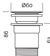
Válvula Pop Down cromo (mm)
