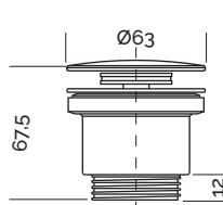
Válvula de salida libre Akron (mm)
